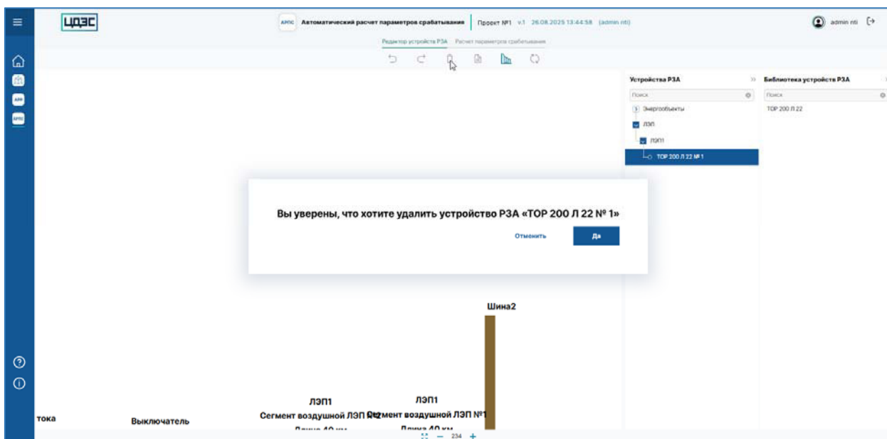
Рисунок 30 – Страница экрана «Редактор устройств РЗА» программного обеспечения «Программный модуль «Автоматизированный расчет параметров срабатывания РЗА»», форма подтверждения удаления пользовательского сценария
