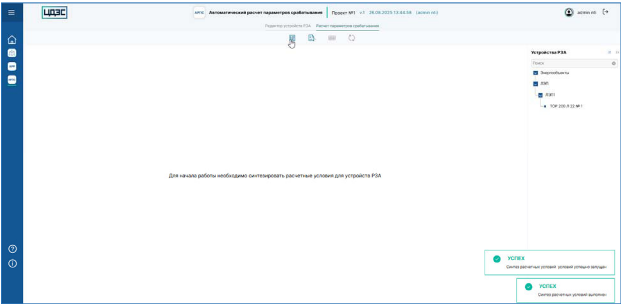
Рисунок 38 – Страница экрана «Расчет параметров срабатывания» программного обеспечения «Программный модуль «Автоматизированный расчет параметров срабатывания РЗА»», синтез расчетных условий функций РЗА выбранных устройств РЗА
