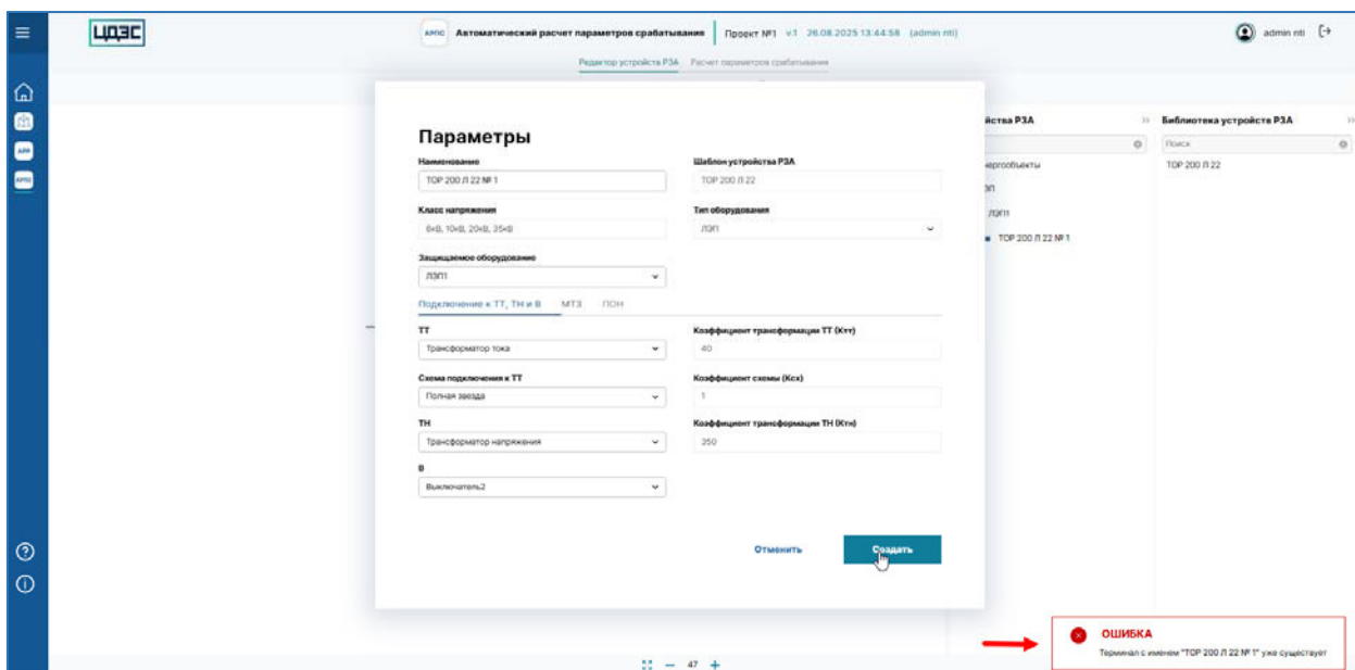
Рисунок 25 – Страница экрана «Редактор устройств РЗА» программного обеспечения «Программный модуль «Автоматизированный расчет параметров срабатывания РЗА»», инициирование создание устройства РЗА с неуникальным наименованием
