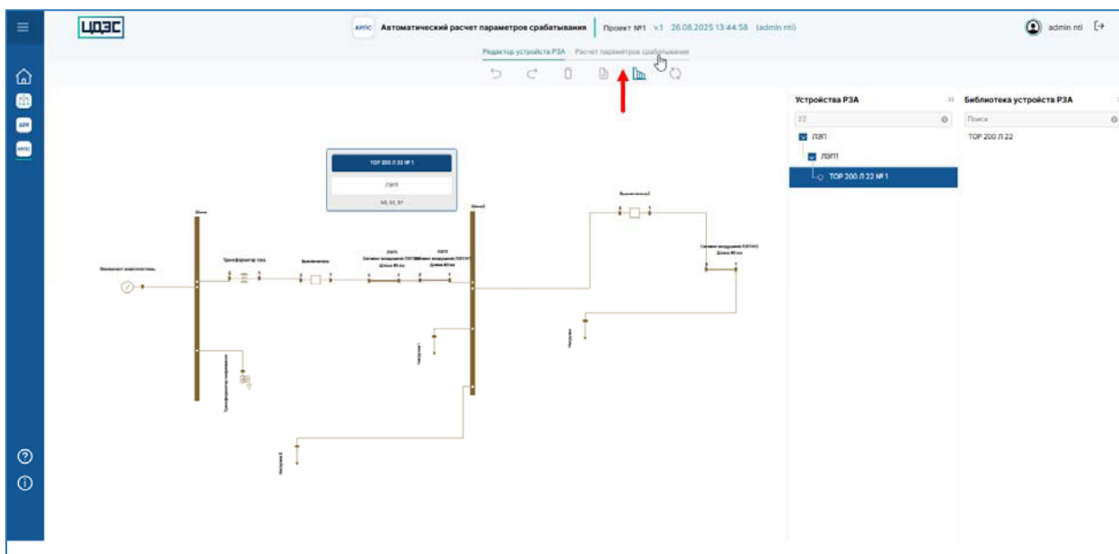
Рисунок 32 – Страница экрана «Редактор устройств РЗА» программного обеспечения «Программный модуль «Автоматизированный расчет параметров срабатывания РЗА»», переход на экран «Расчет параметров срабатывания»
