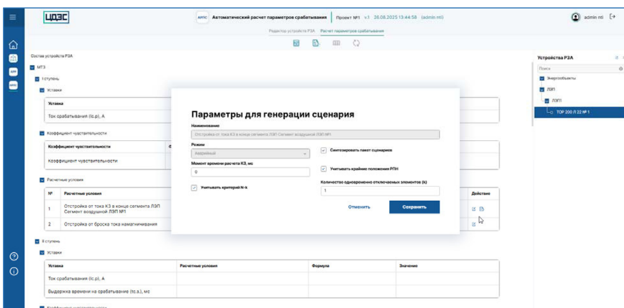
Рисунок 47 – Страница экрана «Расчет параметров срабатывания» программного обеспечения «Программный модуль «Автоматизированный расчет параметров срабатывания РЗА»», форма редактирования параметров сценария расчетного условия функции РЗА выбранного устройства РЗА
