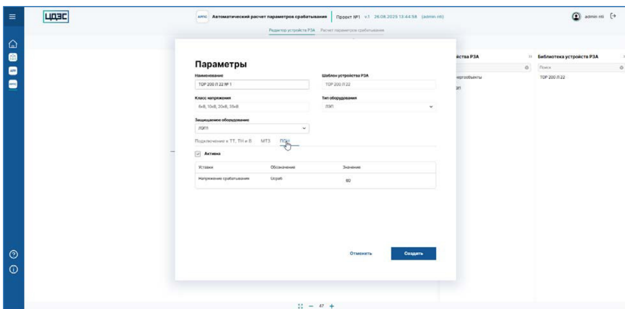
Рисунок 23 – Страница экрана «Редактор устройств РЗА» программного обеспечения «Программный модуль «Автоматизированный расчет параметров срабатывания РЗА»», вкладка «ПОН» формы создания устройства РЗА
