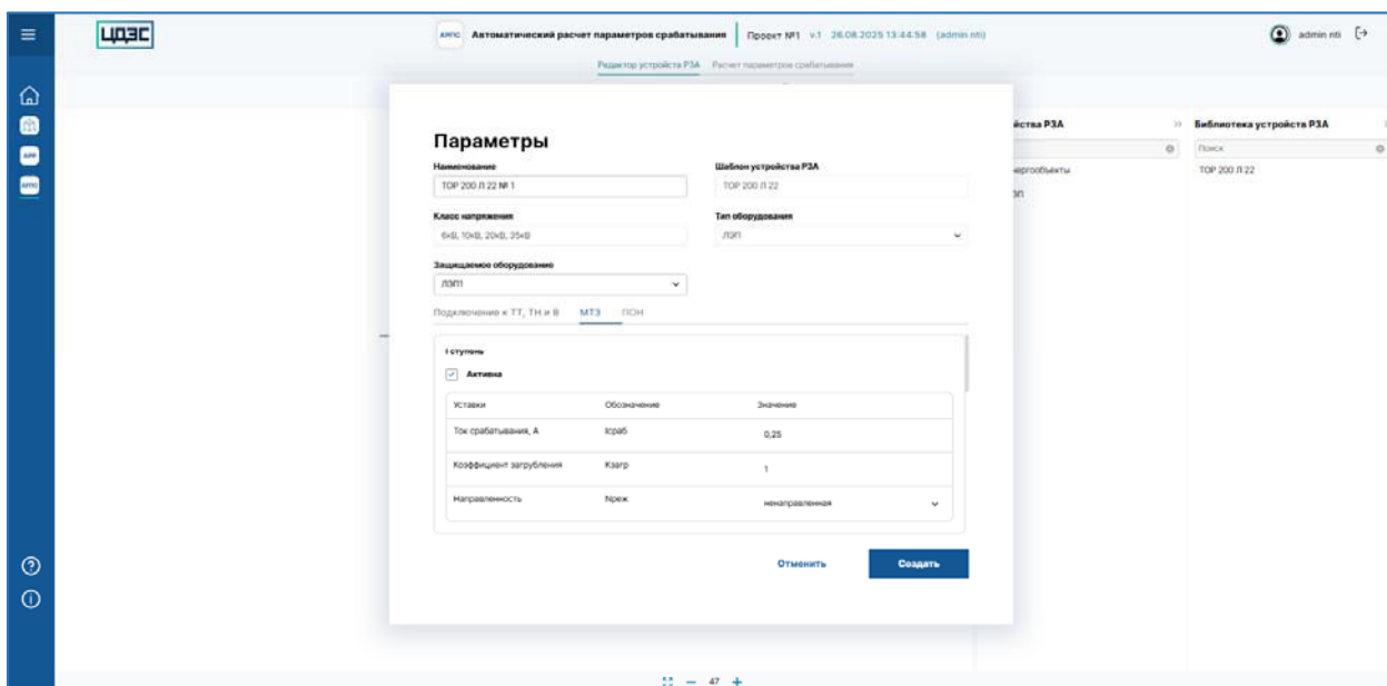
Рисунок 21 – Страница экрана «Редактор устройств РЗА» программного обеспечения «Программный модуль «Автоматизированный расчет параметров срабатывания РЗА»», вкладка «MT3» формы создания устройства РЗА
