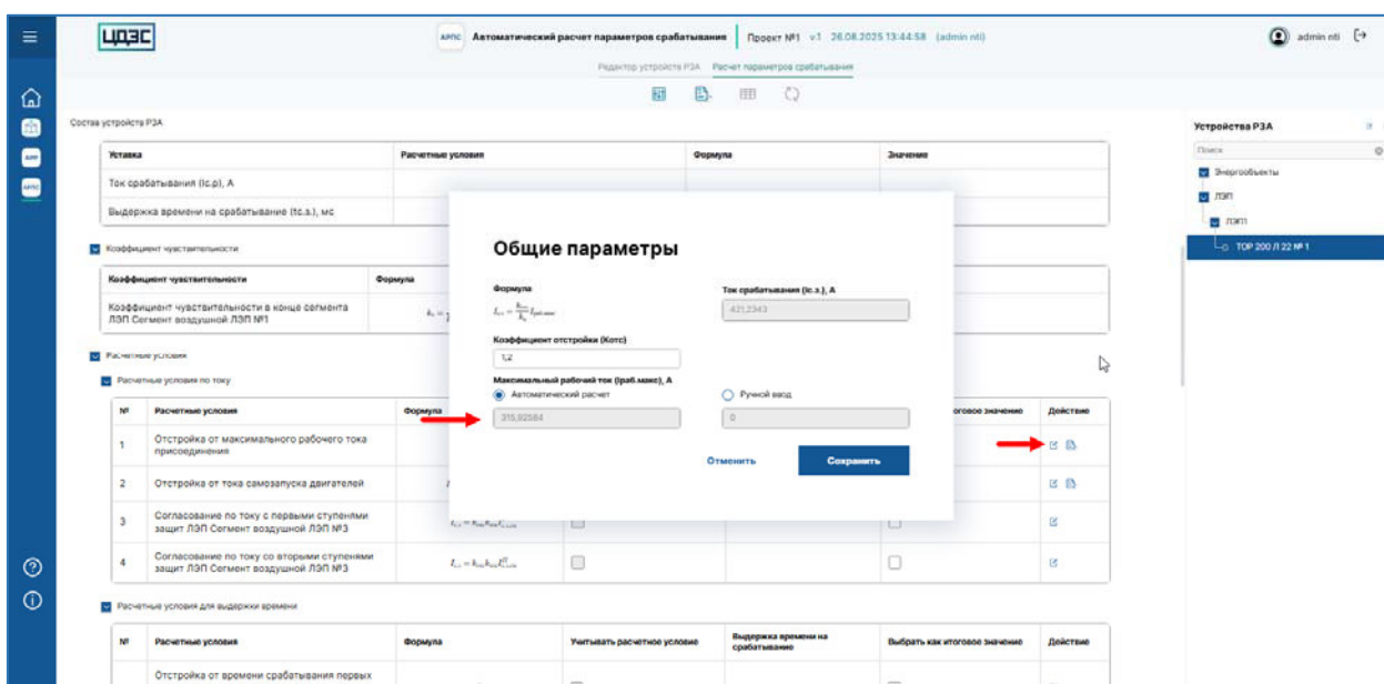
Рисунок 50 – Страница экрана «Расчет параметров срабатывания» программного обеспечения «Программный модуль «Автоматизированный расчет параметров срабатывания РЗА»», просмотр результатов генерации сценариев на основании расчетных условий функций РЗА выбранного устройства РЗА в программном обеспечении «Программный модуль «Автоматизированный расчет режимов»
