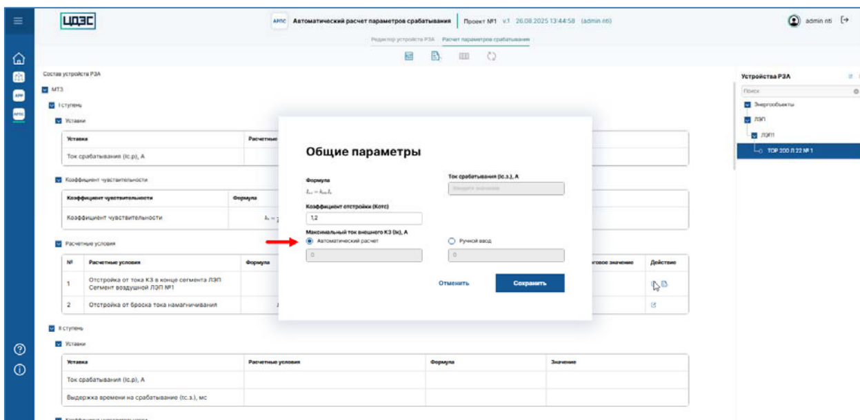
Рисунок 44 – Страница экрана «Расчет параметров срабатывания» программного обеспечения «Программный модуль «Автоматизированный расчет параметров срабатывания РЗА»», форма редактирования параметров расчетного условия функции РЗА выбранного устройства РЗА, где для флага «Учитывать расчетное условие» установлено значение «истина», ввод значений для расчета параметра срабатывания
