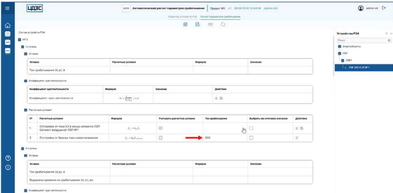
Рисунок 43 – Страница экрана «Расчет параметров срабатывания» программного обеспечения «Программный модуль «Автоматизированный расчет параметров срабатывания РЗА»», рассчитанное значение параметра срабатывания расчетного условия
