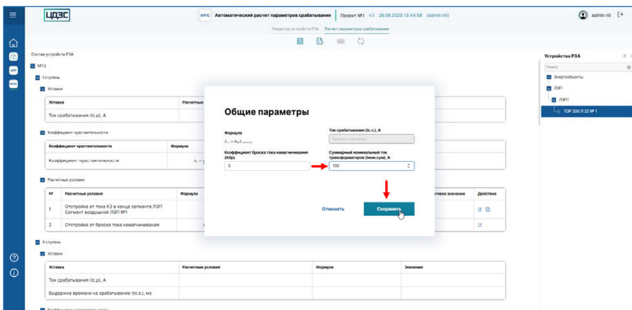
Рисунок 42 – Страница экрана «Расчет параметров срабатывания» программного обеспечения «Программный модуль «Автоматизированный расчет параметров срабатывания РЗА»», форма редактирования параметров расчетного условия функции РЗА выбранного устройства РЗА, где для флага «Учитывать расчетное условие» установлено значение «ложь», ввод значений для расчета параметра срабатывания
