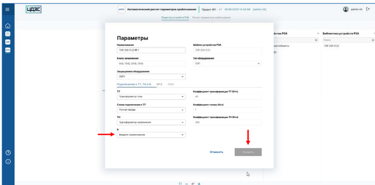
Рисунок 24 – Страница экрана «Редактор устройств РЗА» программного обеспечения «Программный модуль «Автоматизированный расчет параметров срабатывания РЗА»», форма создания устройства РЗА при незаполненном обязательном параметре
