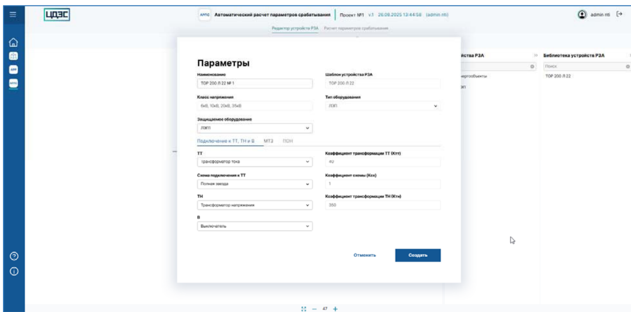
Рисунок 20 – Страница экрана «Редактор устройств РЗА» программного обеспечения «Программный модуль «Автоматизированный расчет параметров срабатывания РЗА»», вкладка «Подключение в ТТ, ТН и В» формы создания устройства РЗА
