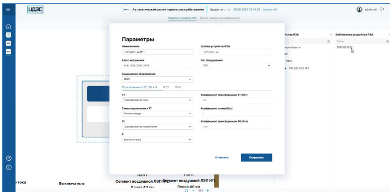
Рисунок 28– Страница экрана «Редактор устройств РЗА» программного обеспечения «Программный модуль «Автоматизированный расчет параметров срабатывания РЗА»», форма редактирования устройства РЗА
