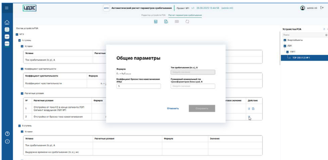
Рисунок 41 – Страница экрана «Расчет параметров срабатывания» программного обеспечения «Программный модуль «Автоматизированный расчет параметров срабатывания РЗА»», форма редактирования параметров расчетного условия функции РЗА выбранного устройства РЗА, где для флага «Учитывать расчетное условие» установлено значение «ложь»
