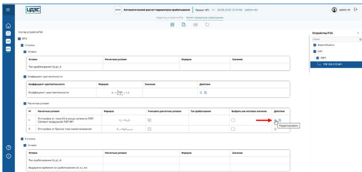
Рисунок 40 – Страница экрана «Расчет параметров срабатывания» программного обеспечения «Программный модуль «Автоматизированный расчет параметров срабатывания РЗА»», инициирование редактирования параметров расчетного условия функции РЗА выбранного устройства РЗА
