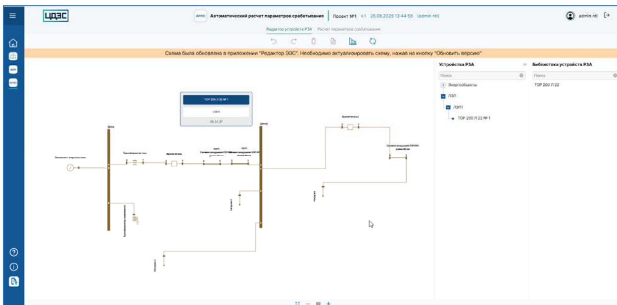
Рисунок 53 – Страница экрана «Расчет параметров срабатывания» программного обеспечения «Программный модуль «Автоматизированный расчет параметров срабатывания РЗА»», вывод информационного сообщения о необходимости обновления версии схемы информационной модели проекта
