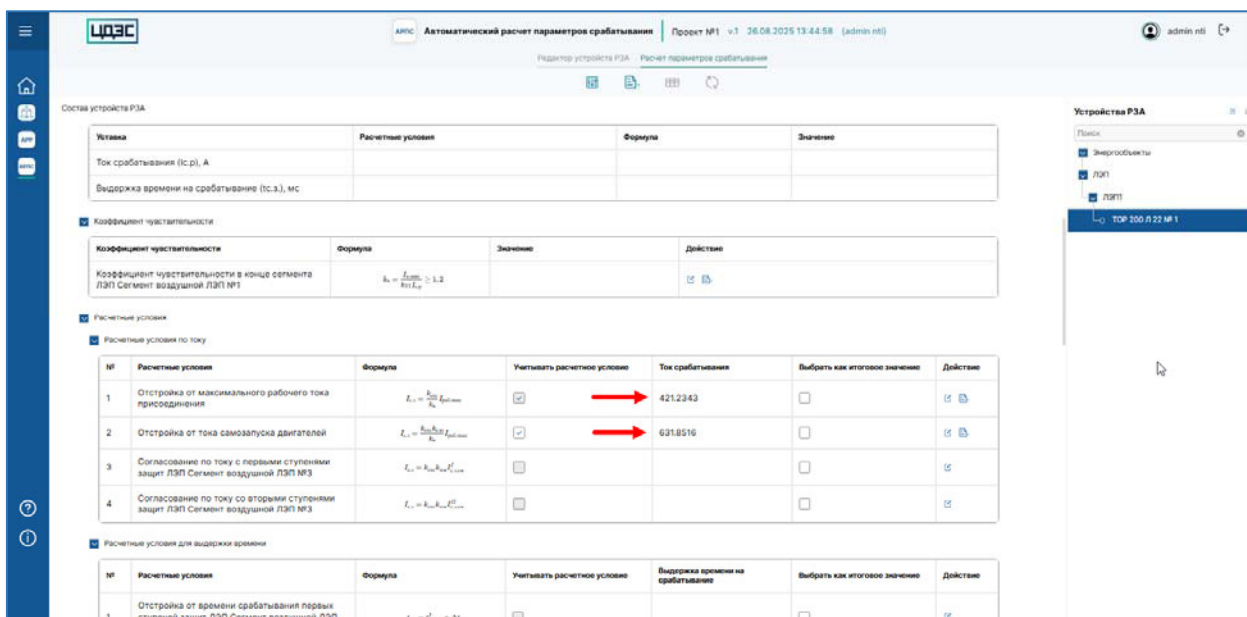
Рисунок 49 – Страница экрана «Расчет параметров срабатывания» программного обеспечения «Программный модуль «Автоматизированный расчет параметров срабатывания РЗА»», результат генерации сценариев на основании расчетных условий функций РЗА выбранного устройства РЗА в программном обеспечении «Программный модуль «Автоматизированный расчет режимов»
