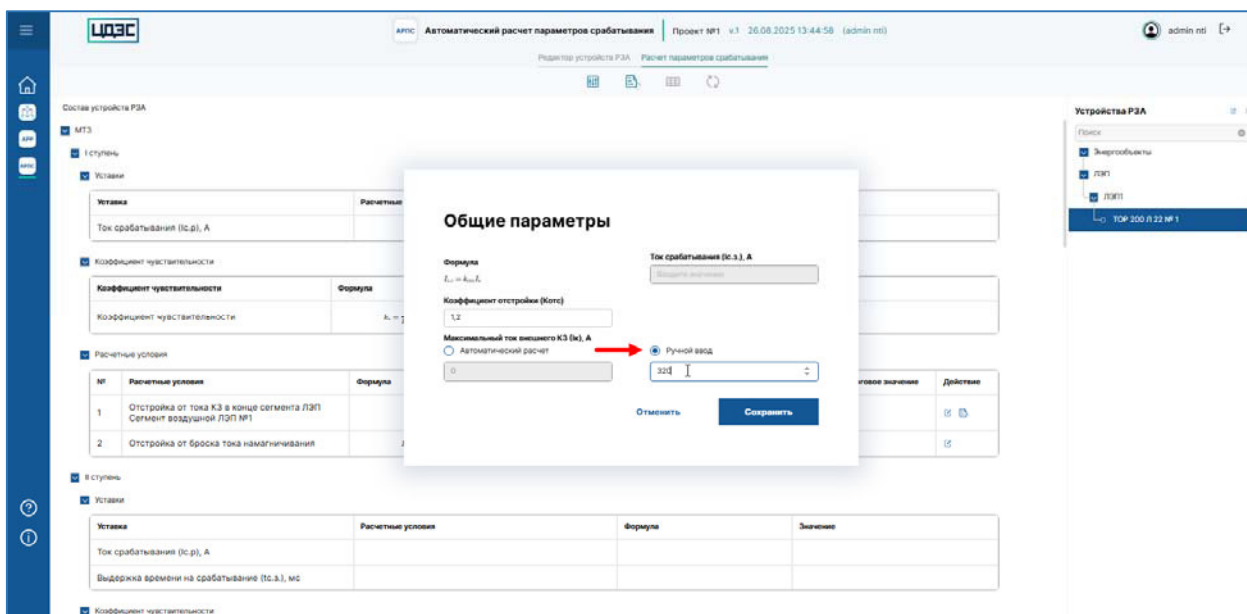
Рисунок 45 – Страница экрана «Расчет параметров срабатывания» программного обеспечения «Программный модуль «Автоматизированный расчет параметров срабатывания РЗА»», форма редактирования параметров расчетного условия функции РЗА выбранного устройства РЗА, ввод значений для расчета параметра срабатывания
