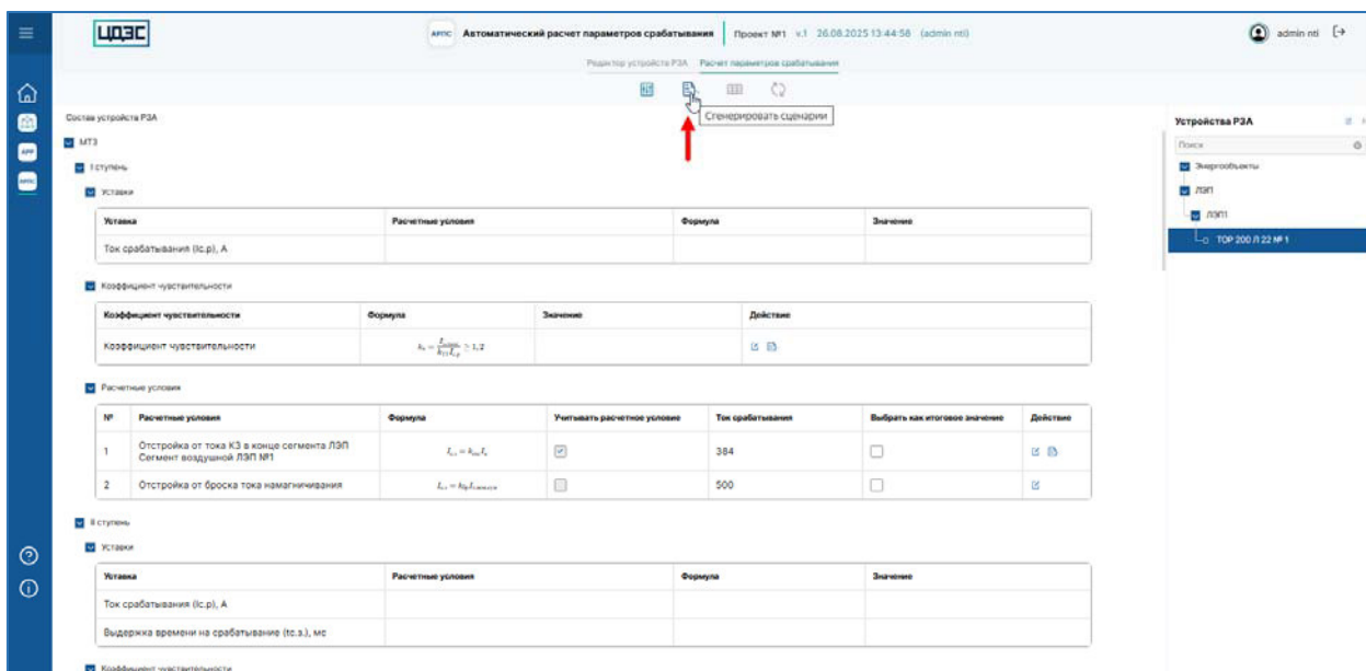
Рисунок 48 – Страница экрана «Расчет параметров срабатывания» программного обеспечения «Программный модуль «Автоматизированный расчет параметров срабатывания РЗА»», инициирование генерации сценариев на основании расчетных условий функций РЗА выбранного устройства РЗА в программном обеспечении «Программный модуль «Автоматизированный расчет режимов»»
