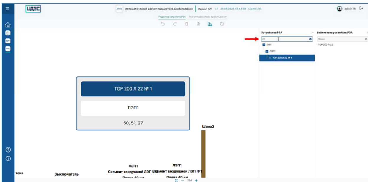
Рисунок 31 – Страница экрана «Редактор устройств РЗА» программного обеспечения «Программный модуль «Автоматизированный расчет параметров срабатывания РЗА»», работа со списком устройств РЗА
