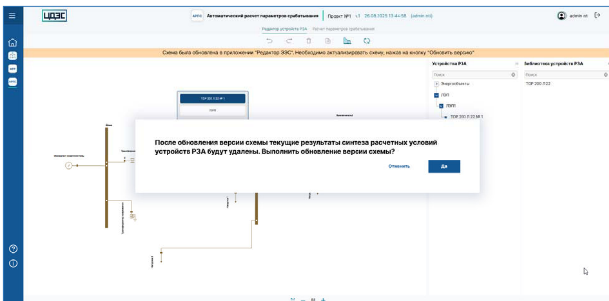
Рисунок 55 – Страница экрана «Редактор устройств РЗА» программного обеспечения «Программный модуль «Автоматизированный расчет параметров срабатывания РЗА»», подтверждение обновления версии схемы информационной модели проекта
