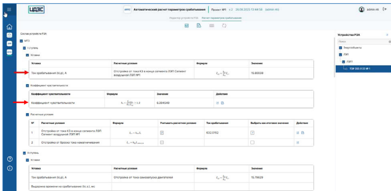
Рисунок 52 – Страница экрана «Расчет параметров срабатывания» программного обеспечения «Программный модуль «Автоматизированный расчет параметров срабатывания РЗА»», итоговые значения параметра срабатывания и коэффициента чувствительности функций РЗА выбранного устройства РЗА
