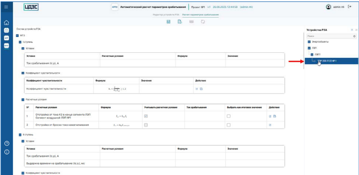
Рисунок 39 – Страница экрана «Расчет параметров срабатывания» программного обеспечения «Программный модуль «Автоматизированный расчет параметров срабатывания РЗА»», состав расчетных условий функций РЗА выбранного устройства РЗА
